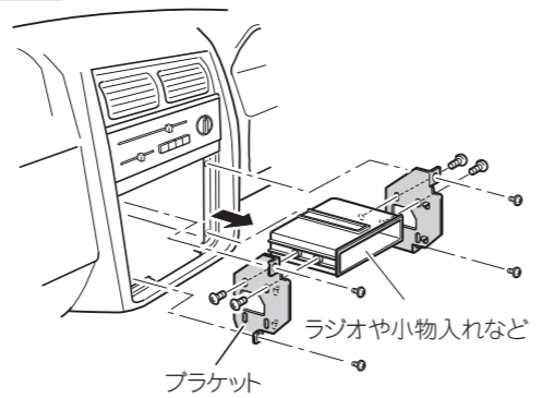
ブラケット
