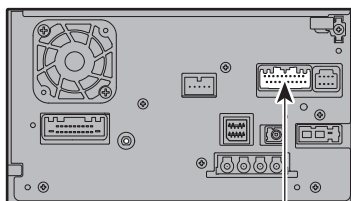
ナビゲーション本体 (例:AVIC-EVZ9)
