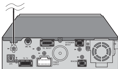
DVD/CD ユニット内蔵 HDD ナビゲーションサーバー 「AVIC-H09」
