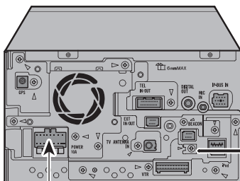
電源コード 黒
