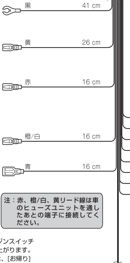
電源コード
