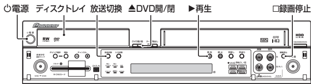
DVR-RT900D(ドアを開いた状態)
