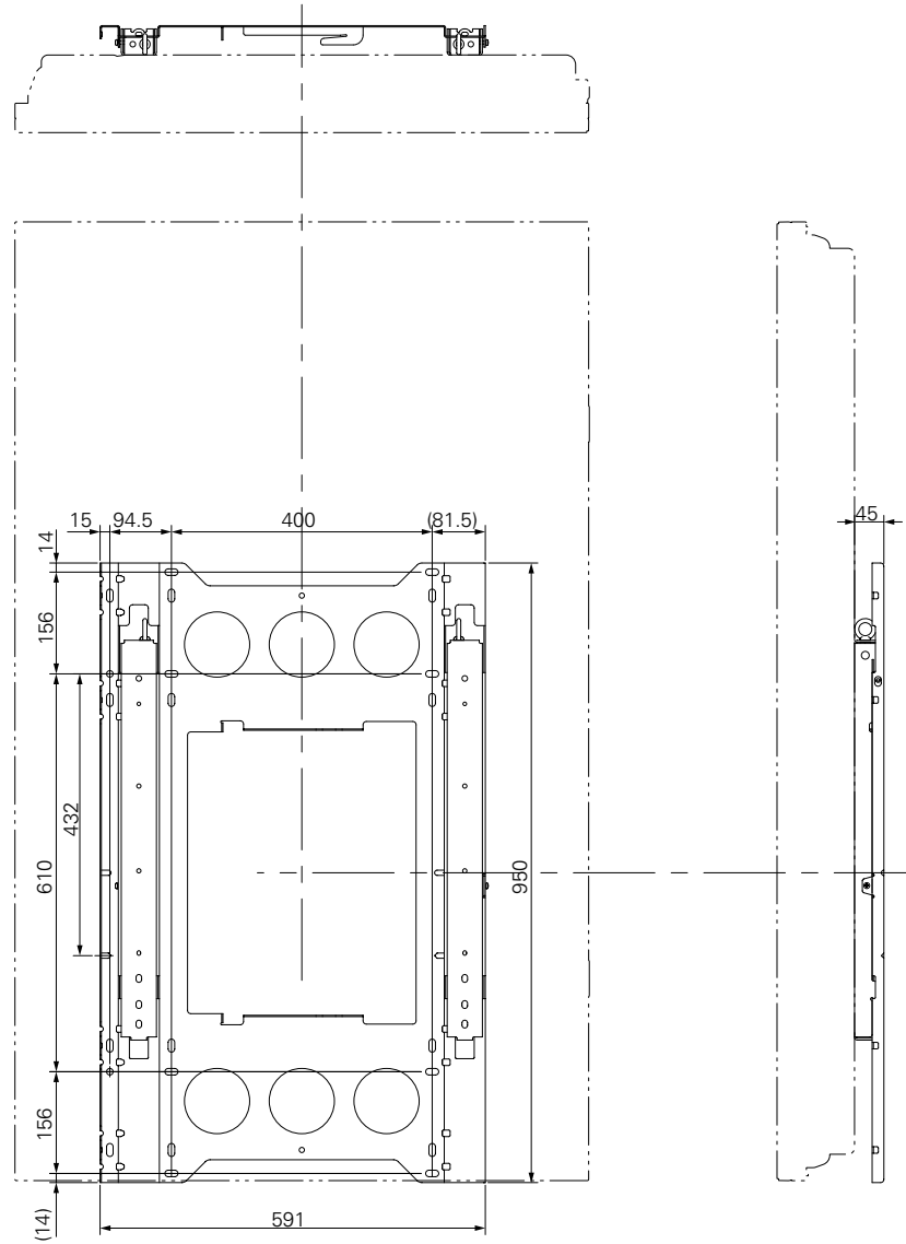
寸法図 (単位：mm)
