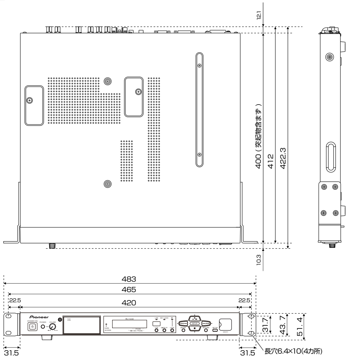
寸法図 (単位:mm)
